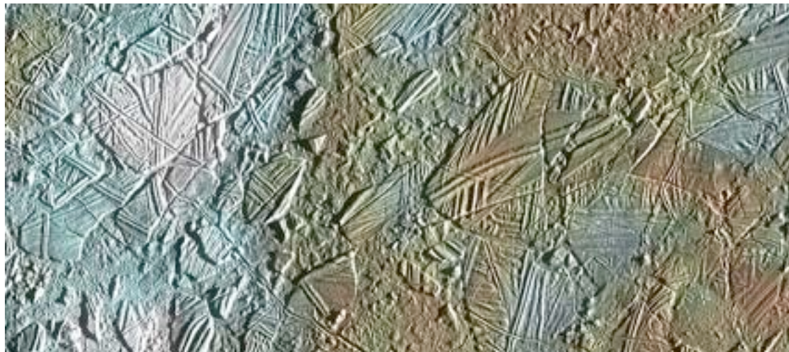
Conamara Chaos
