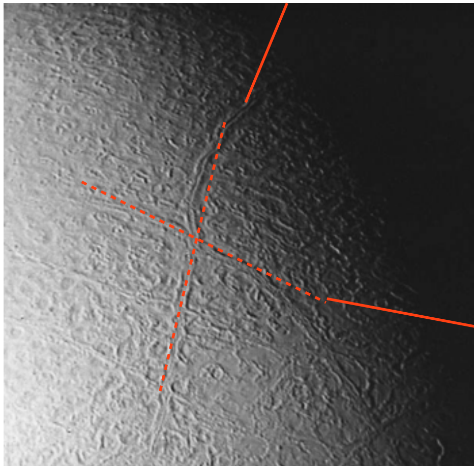
Tano Sulci
