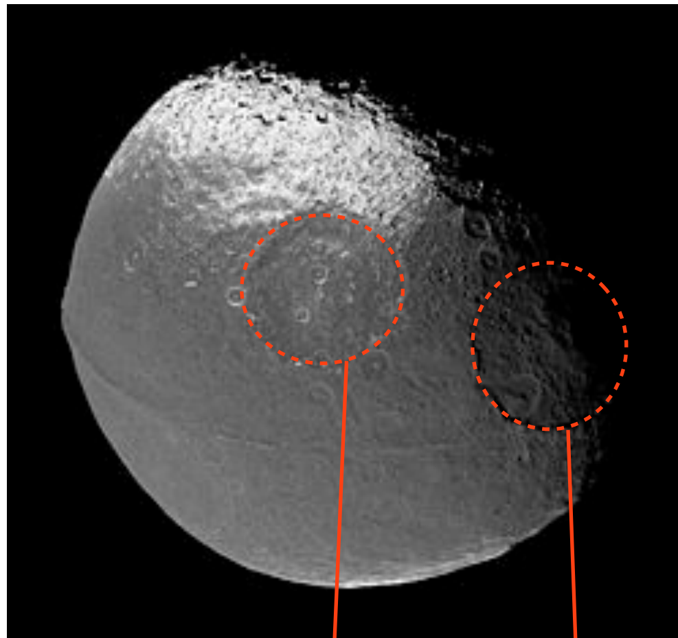
Falsaron
