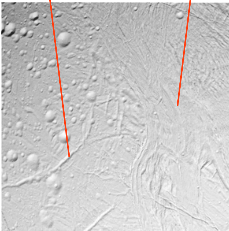
Samarkand Sulci
