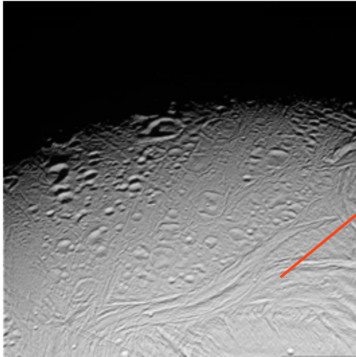
Samarkand Sulci
