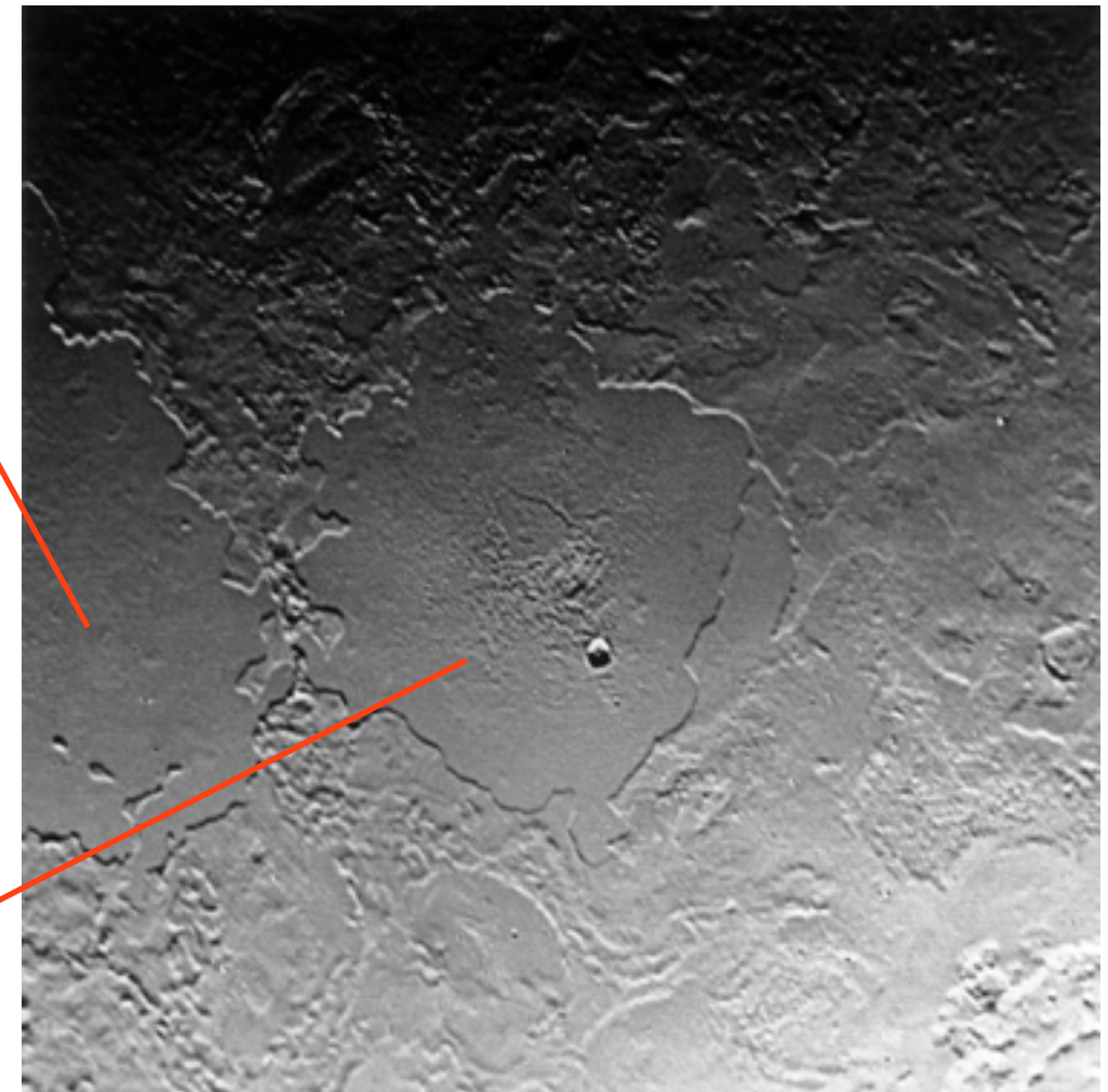
Tuonela Planitia
